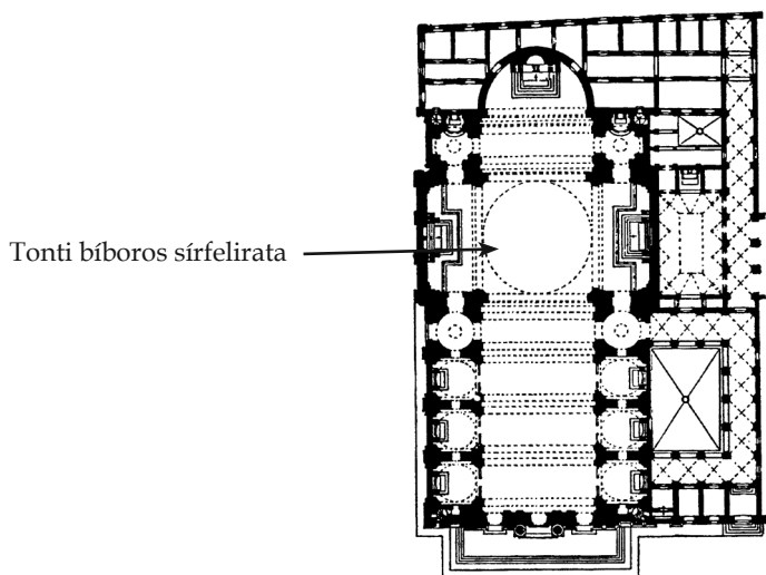
Az II Gesù-templom alaprajza
