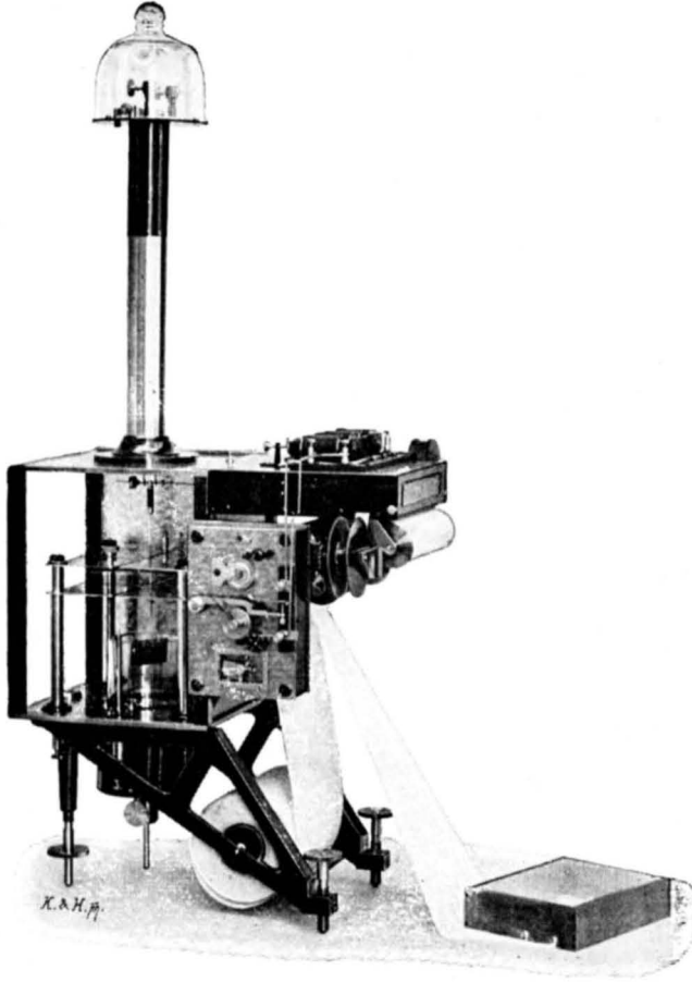
Benndorf-féle elektromos regisztrator.
