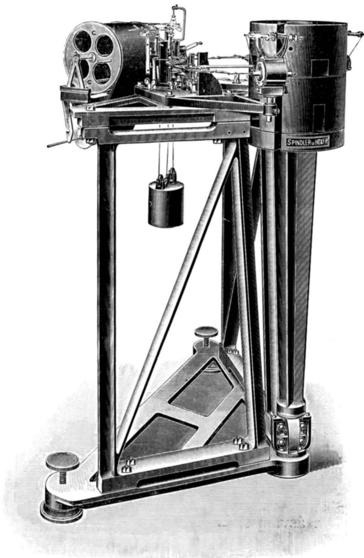
Wichert-féle elektromos földrengésmutató (Seismograph).
